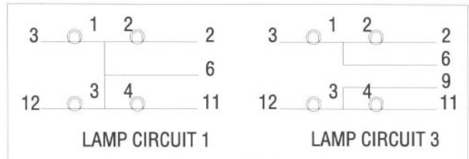
Lamp Circuits
